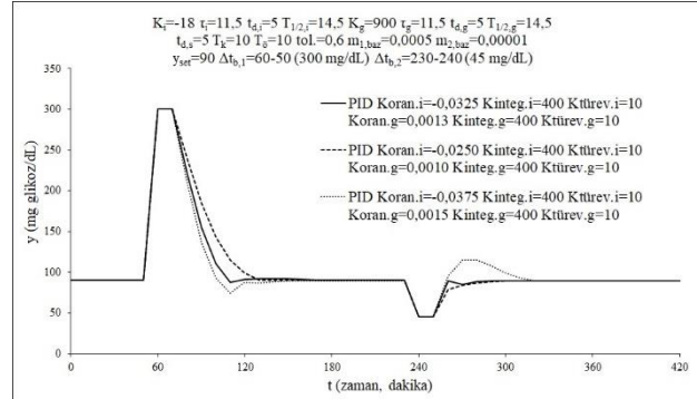
Şekil 4.2.a. PID denetleyici performansı üzerindeki oransal denetçi kazancı etkisi. Karşılaştırmalı olarak zamana karşı ikinci girdi (plazma glikoz seviyesi) grafiği. İnsülin kazancı ( K_i ) = -18 mg glikoz/U; insülin zaman sabiti ( \tau_i ) = 11,5 dakika; insülin ölü zamanı ( t_{d,i} ) = 5 dakika; insülin yarılanma süresi ( T_{1/2,i} ) = 14,5 dakika; glukagon kazancı ( K_g ) = 900 mg glikoz/U; glukagon zaman sabiti ( \tau_g ) = 11,5 dakika; glukagon ölü zamanı ( t_{d,g} ) = 5 dakika; glukagon yarılanma süresi ( T_{1/2,g} ) = 14,5 dakika; sensör gecikmesi ( t_{d,s} ) = 5 dakika; kontrol aralığı ( T_s ) = 10 dakika; örneklem aralığı ( T_o ) = 10 dakika; insülin açık denge konumu seviyesi ( m_{1,baz} ) = 0,0005 U/dL; glukagon açık denge konumu seviyesi ( m_{2,baz} ) = 0,00001 IU/dL; açlık denge konumu kan şekeri ( y_{set} ) = 90 mg glikoz/dL; açlık denge konumu kan şekeri toleransı (tol.) = \pm 0,6 mg glikoz/dL; birinci bozucu etki süresi ve seviyesi ( \Delta t_{b,1} ) 60-50 dakika ve 300 mg/dL; ikinci bozucu etki süresi ve seviyesi ( \Delta t_{b,2} ) 230-240 dakika ve 45 mg/dL; insülin için integral denetleyici sabiti ( K_{integ.i} ) = 400; insülin için türevsel denetleyici sabiti ( K_{türev.i} ) = 10; glukagon için oransal denetleyici sabiti ( K_{oran.g} ) = 0,0013 veya 0,0010 veya 0,0015; glukagon için integral denetleyici sabiti ( K_{integ.g} ) = 400; glukagon için türevsel denetleyici sabiti ( K_{türev.g} ) = 10.
