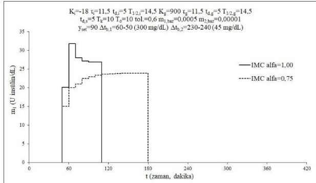
Şekil 4.1.b. IMC denetleyici performansı üzerindeki filtre etkisi. Karşılaştırmalı olarak zamana karşı birinci girdi (insülin) grafiği. İnsülin kazancı ( K_i ) = -18 mg glikoz/U; insülin zaman sabiti ( \tau_i ) = 11,5 dakika; insülin ölü zamanı ( t_{d,i} ) = 5 dakika; insülin yarılanma süresi ( T_{1/2,i} ) = 14,5 dakika; glukagon kazancı ( K_g ) = 900 mg glikoz/U; glukagon zaman sabiti ( \tau_g ) = 11,5 dakika; glukagon ölü zamanı ( t_{d,g} ) = 5 dakika; glukagon yarılanma süresi ( T_{1/2,g} ) = 14,5 dakika; sensör gecikmesi ( t_{d,s} ) = 5 dakika; kontrol aralığı ( T_s ) = 10 dakika; örneklem aralığı ( T_o ) = 10 dakika; insülin açık denge konumu seviyesi ( m_{1,baz} ) = 0,0005 U/dL; glukagon açık denge konumu seviyesi ( m_{2,baz} ) = 0,00001 IU/dL; açlık denge konumu kan şekeri ( y_{set} ) = 90 mg glikoz/dL; açlık denge konumu kan şekeri toleransı (tol.) = \pm 0,6 mg glikoz/dL; birinci bozucu etki süresi ve seviyesi ( \Delta t_{b,1} ) 60-50 dakika ve 300 mg/dL; ikinci bozucu etki süresi ve seviyesi ( \Delta t_{b,2} ) 230-240 dakika ve 45 mg/dL; IMC denetleyici filtre sabiti \alpha (alfa) = 1,00 veya 0,75.
